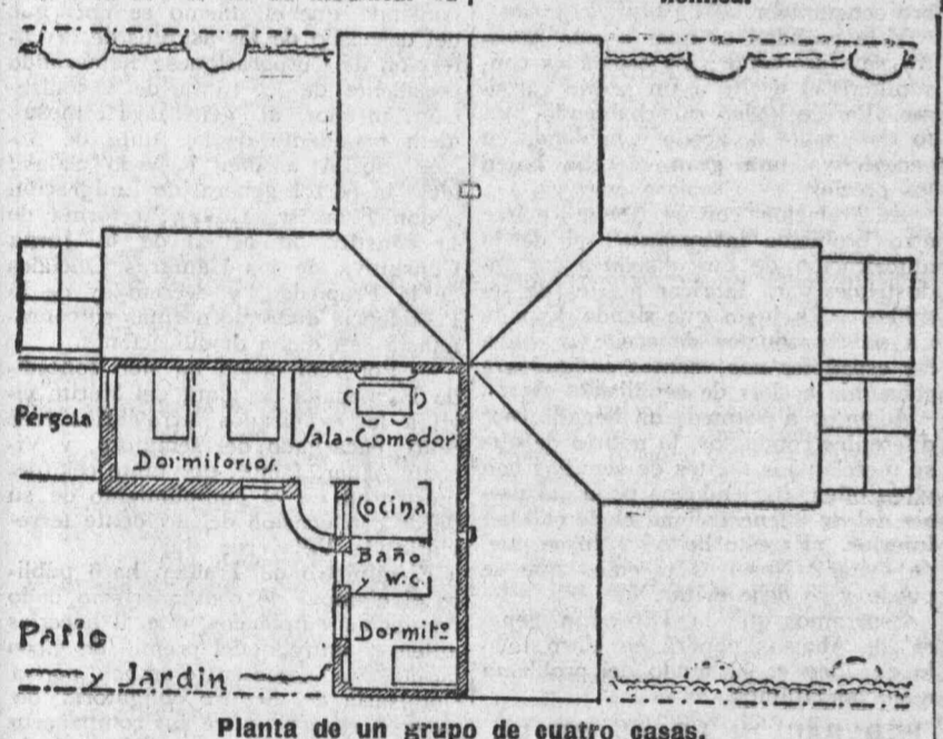
Planta de un grupo de cuatro casas.
