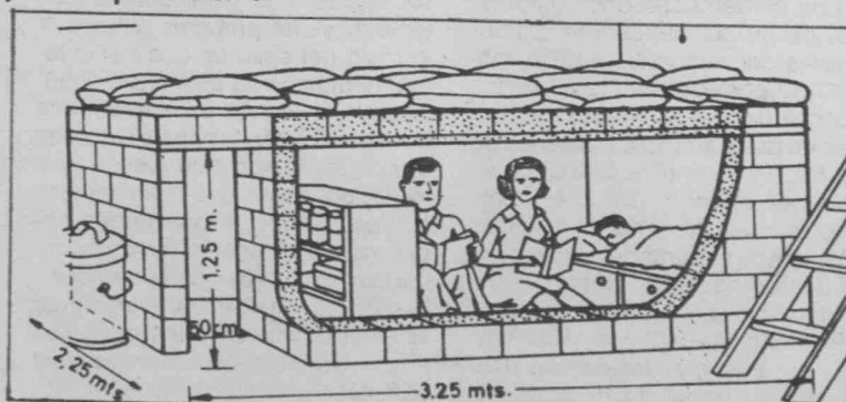
Modelo de refugio familiar para evitar la contaminación radiactiva.
