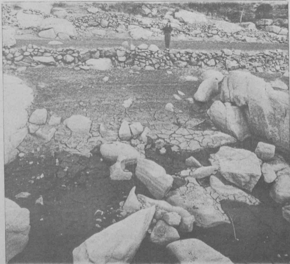
La desertización avanza en toda España. La sequía supuso una parálisis de año y medio en la vida del suelo.
