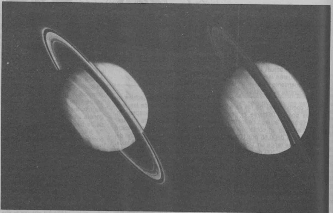
Cien mil anillos rodean al planeta más distinguido del sistema solar.
