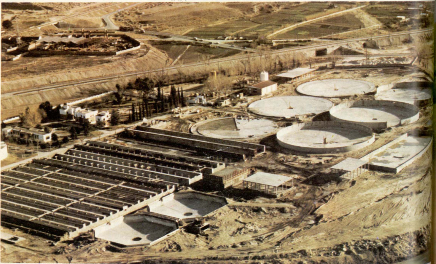
Obras de ampliación de la estación depuradora de aguas residuales «La China», Madrid.
