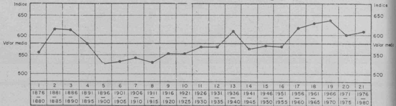
VALORES DEL INDICE DE PLUVIOSIDAD EN LA ESPAÑA PENINSULAR EN CADA UNO DE LOS 21 LUSTROS DEL PERIODO 1876 A 1980
