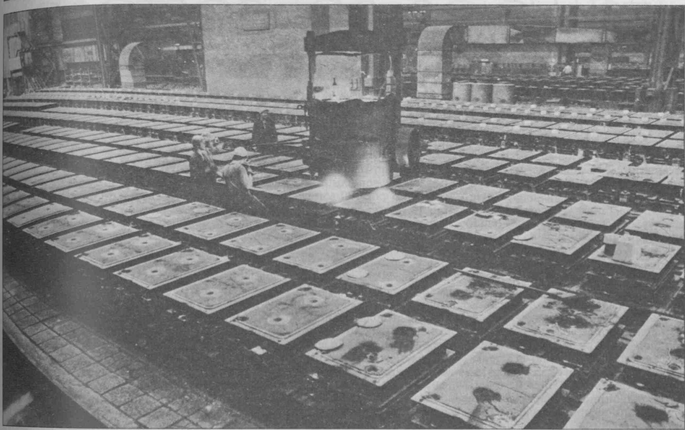
Las instalaciones siderúrgicas alemanas se han acercado a la tecnología japonesa tras la reconversión.
