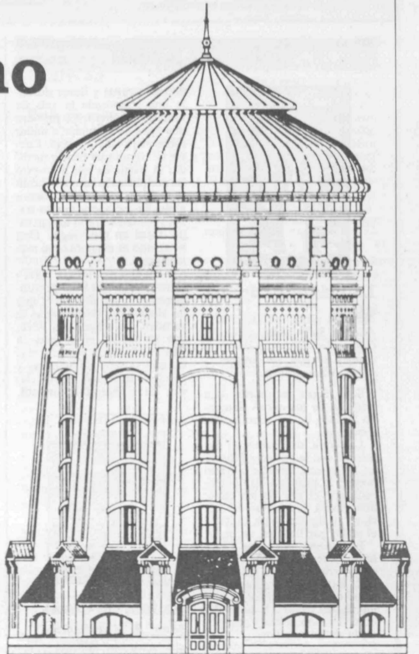
Alzado del primer depósito elevado del Canal de Isabel II después de su recuperación.
