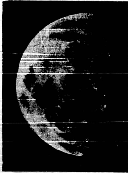
Una magnífica fotografía de la Luna, obtenida por el Observatorio Astronómico de Madrid.
